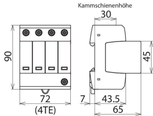
Maßbild VT2 M TT 320 AT
