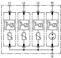
Prinzipialschaltbild VT2 M TT 320 AT
