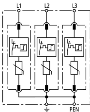
Prinzipschaltbild VT2 M TNC 320 AT
