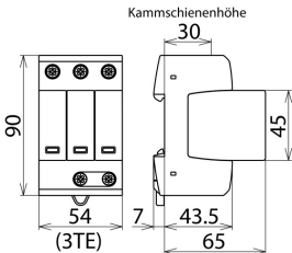
Maßbild VT2 M TNC 320 AT
