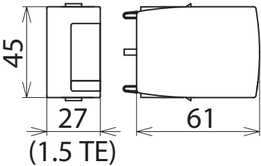
Maßbild
