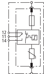
Prinzipschaltbild
