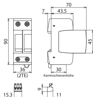
Maßbild
