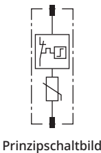
Prinzipschaltbild
