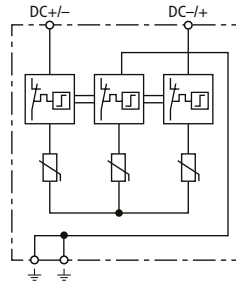
Prinzipschaltbild
