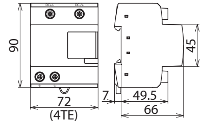
Maßbild
