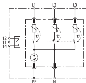
Prinzipschaltbild
