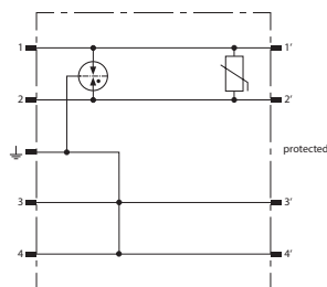
Prinzipschaltbild
