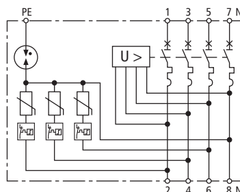
Prinzipschaltbild
