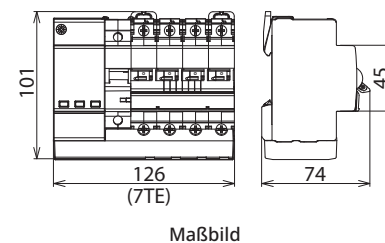
Maßbild
