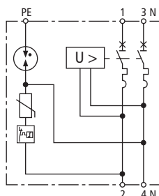
Prinzipschaltbild
