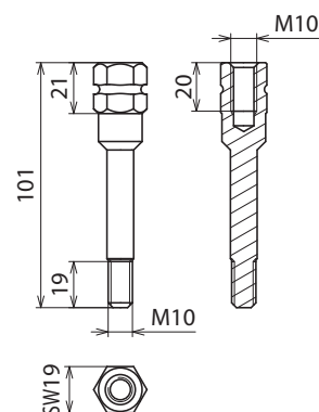
Maßbild
