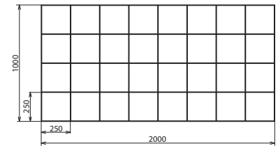
Maßbild
