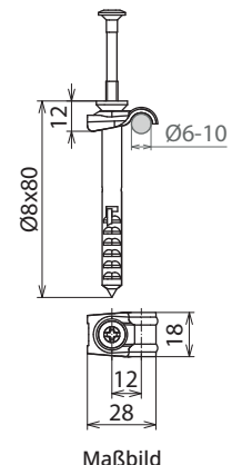
Maßbild
