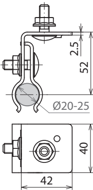
Maßbild
