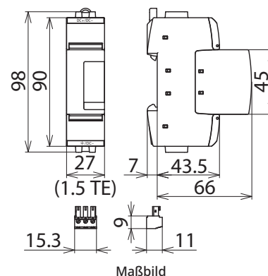
Maßbild
