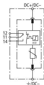
Prinzipschaltbild
