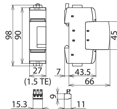
Maßbild
