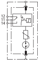
Prinzipschaltbild
