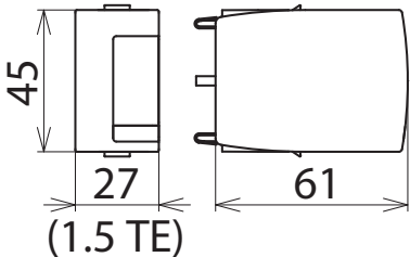
Maßbild
