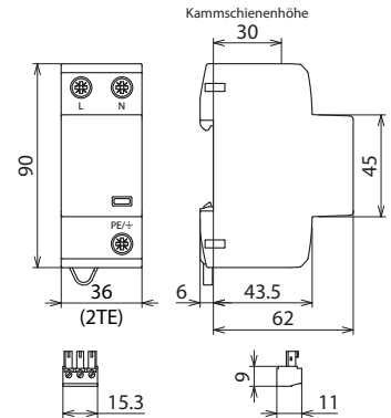
Maßbild
