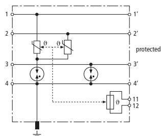
Prinzipschaltbild
