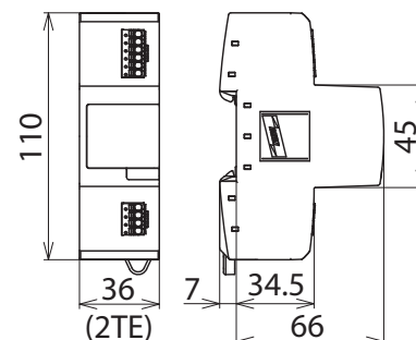
Maßbild
