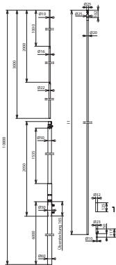
Maßbild
