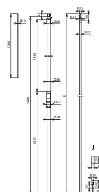
Maßbild
