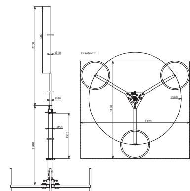
Maßbild
