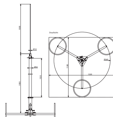
Maßbild
