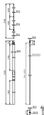
Maßbild
