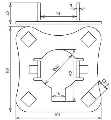
Maßbild
