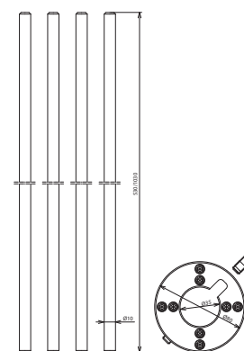
Maßbild
