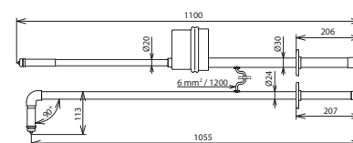
Maßbild
