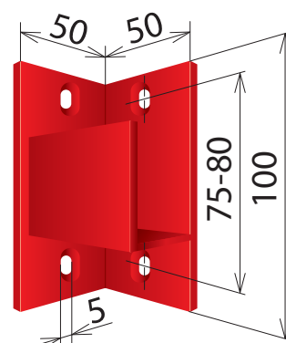
Maßbild
