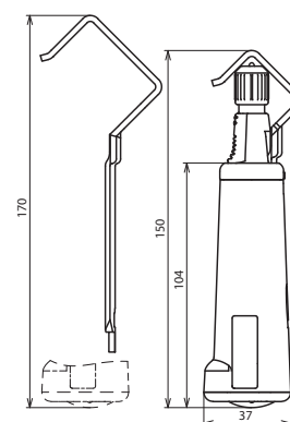
Maßbild
