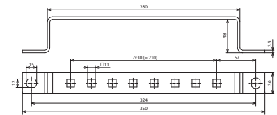
Maßbild
