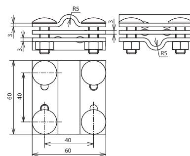
Maßbild
