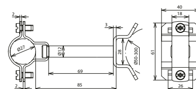
Maßbild
