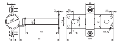
Maßbild
