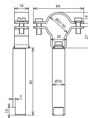
Maßbild
