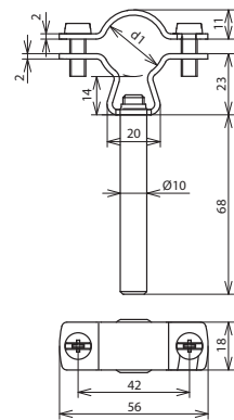
Maßbild
