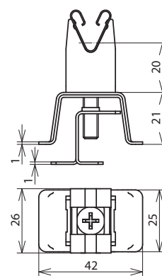
Maßbild
