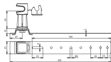
Maßbild
