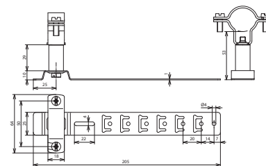
Maßbild
