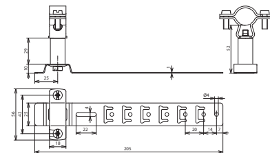
Maßbild
