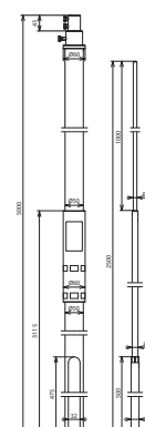
Maßbild
