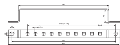
Maßbild
