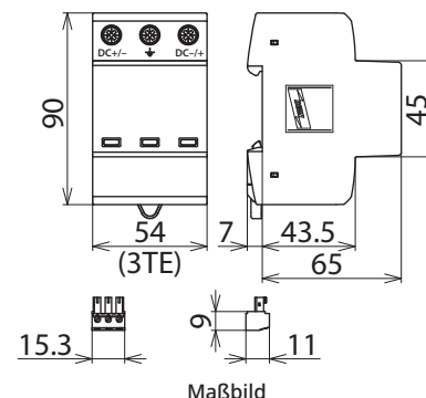
Maßbild
