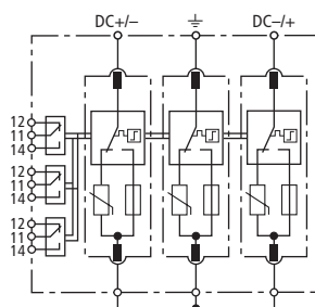
Prinzipschaltbild
