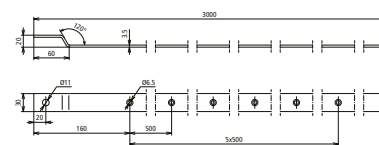
Maßbild
