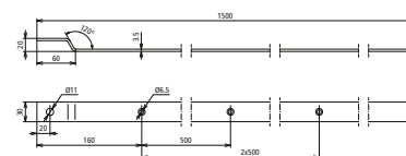
Maßbild
