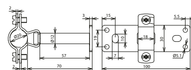
Maßbild
