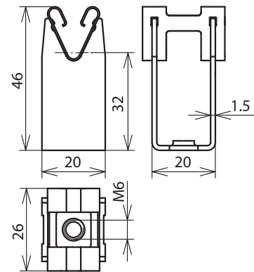
Maßbild
