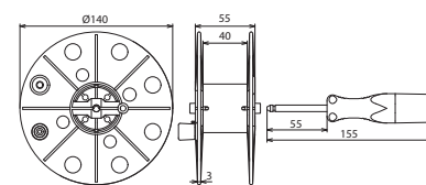
Maßbild
