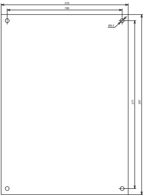
Maßbild
